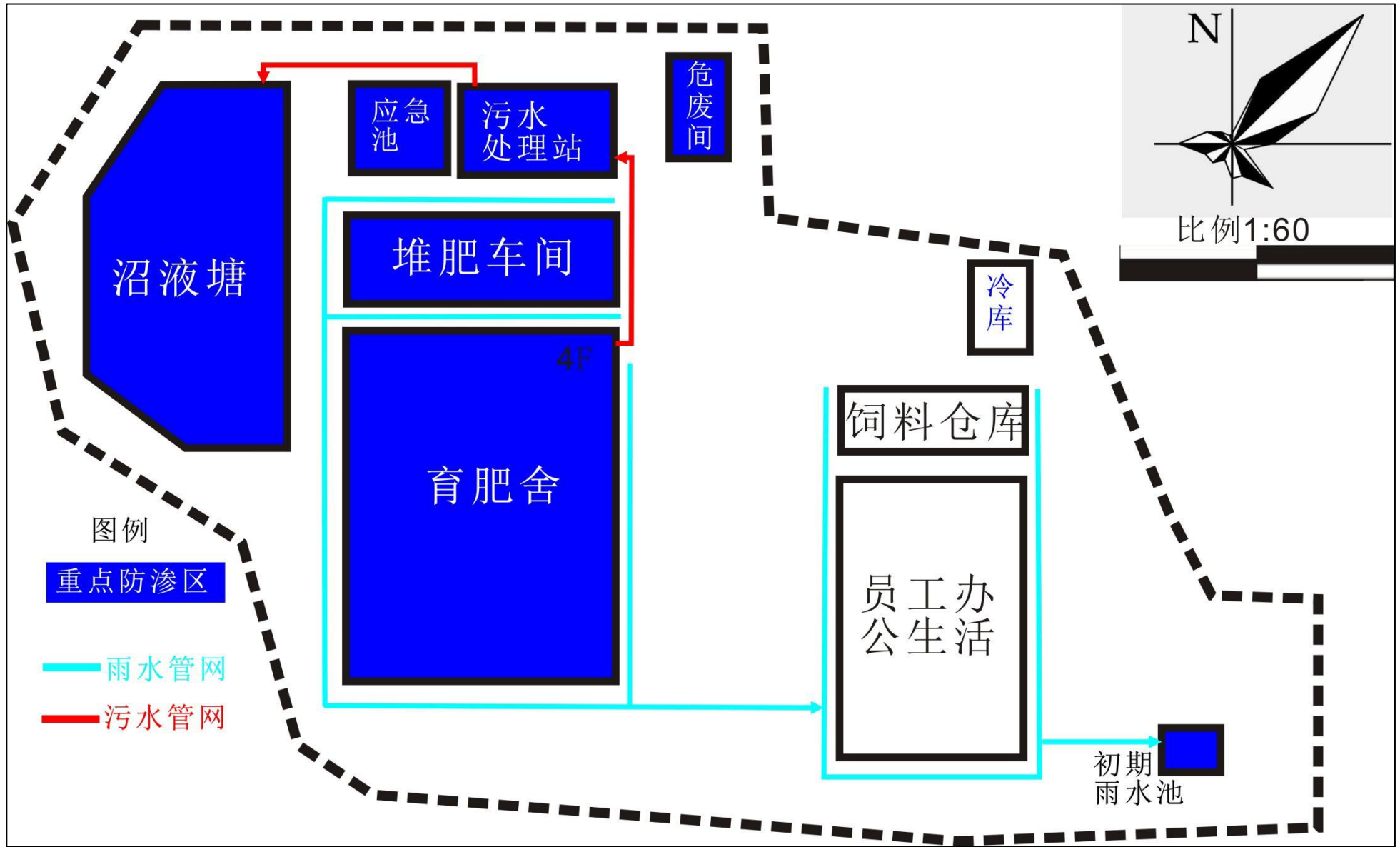
附图6 项目雨污管网及重点防渗图
